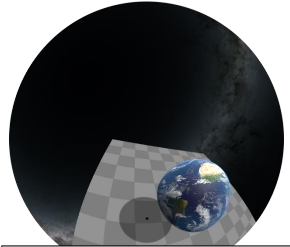
Sonnenfinsternis 29.05.1919
