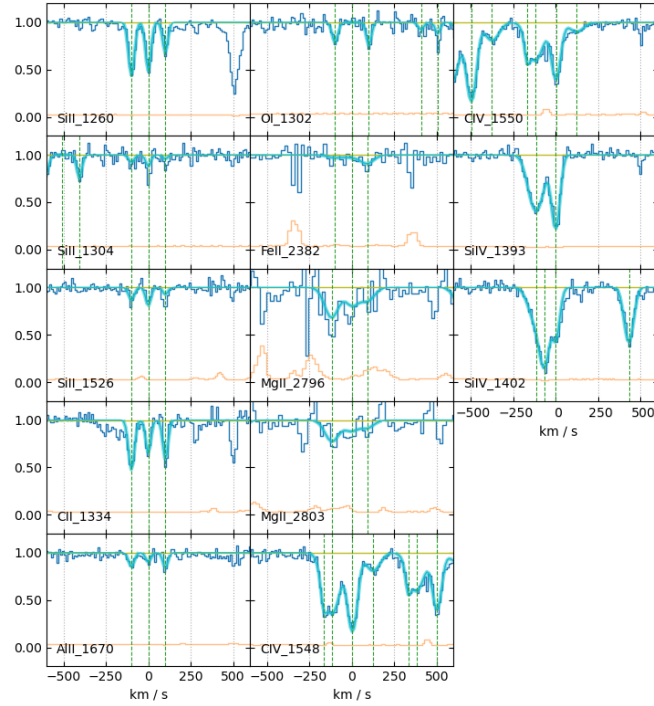
J0247-0556 z4.13952
