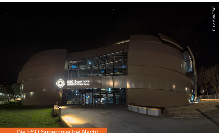
Die ESO Supernova bei Nacht
